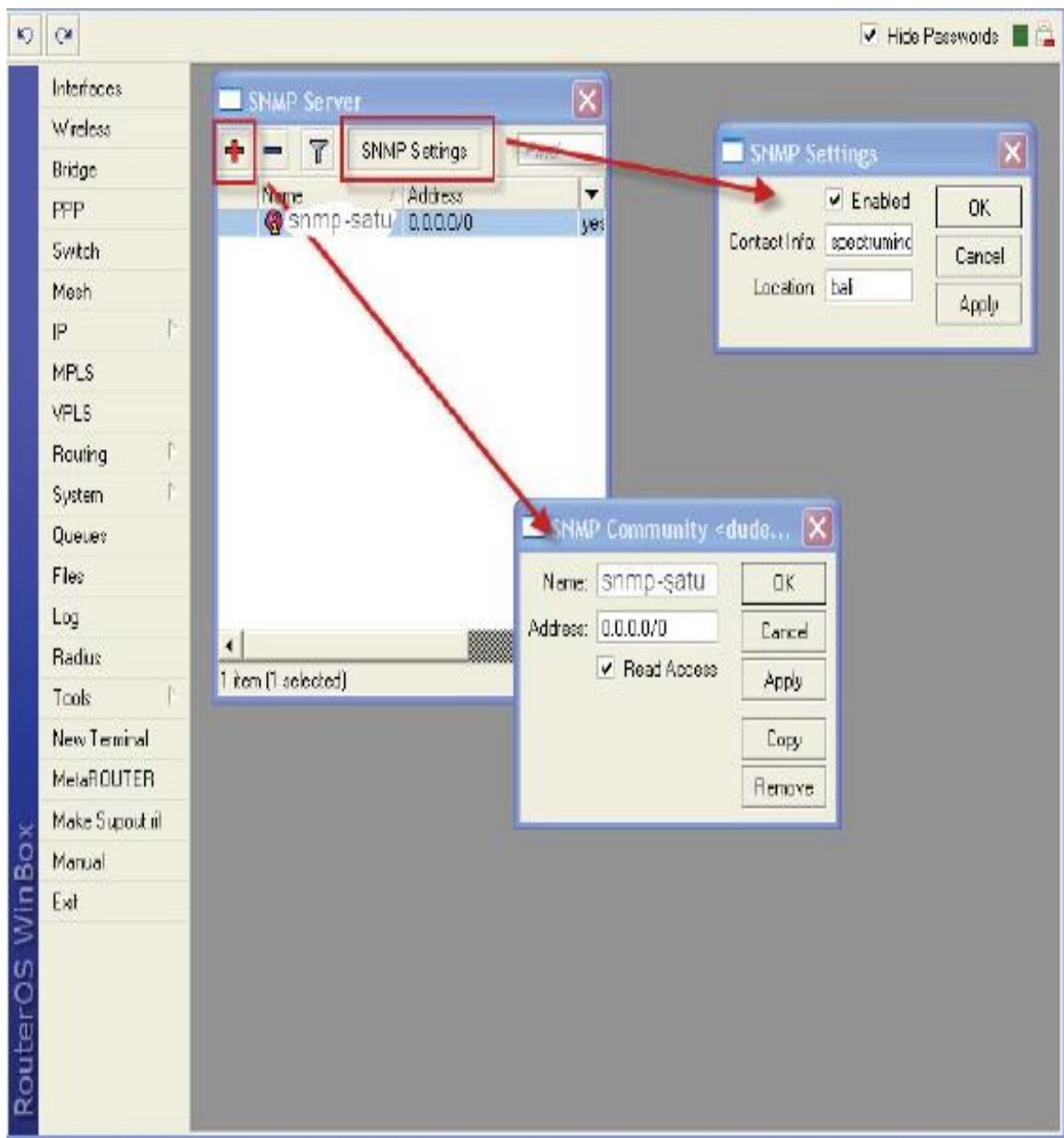
Gambar 5. Pengaturan IP SNMP
