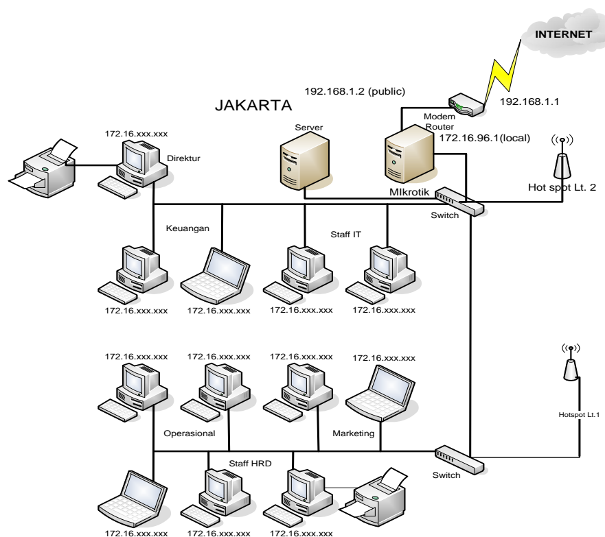
Gambar 4. Skema rancangan jaringan usulan.
